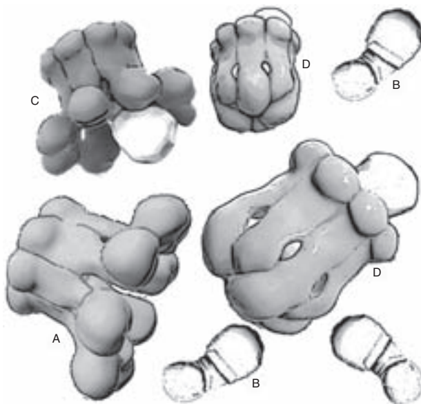
Slika 1. Molekule sugamadeksa (A) zbog lipofilnosti svojoj unutrašnjoj šupljini privlače molekule rokuronija (B) te s njima formiraju stabilne komplekse (C i D) koji se nepromijenjeni izlučuju putem bubrega.
